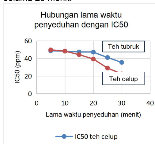
Gambar 1. Grafik hubungan antara lama waktu penyeduhan dengan IC 50 .
